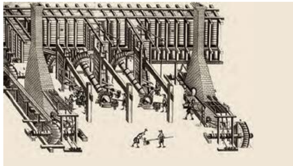
Молотовые станы, употреблявшиеся на заводах Урала. Из альбома И.А. Шлаттера, 1760 год
