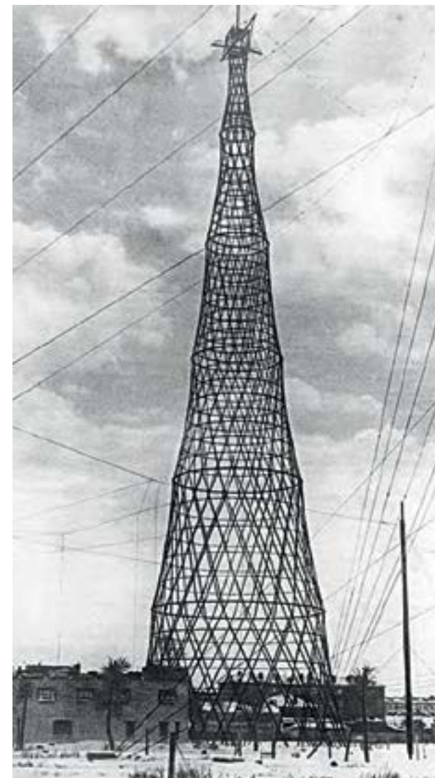
Башня телевизионного центра на Шаболовке конструкции В.Г. Шухова. Фото, 1940-е годы
